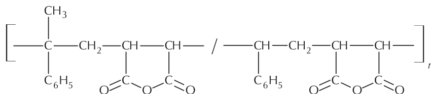
poli[(izopropenilbenzen;stiren)-alt-maleinanhidrid]
