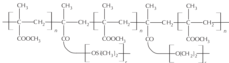
poli(metil-metakrilat)-graft-[poli(dimetilsiloksan);poli(oksiran)]
