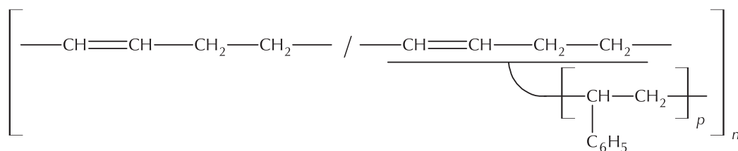
poli(buta-1,3-dien)-tris(graft-polistiren) a
