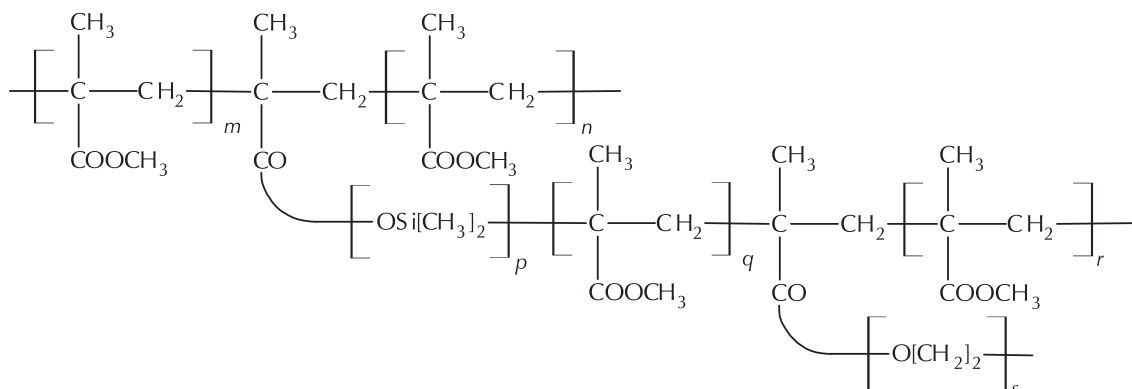
poli(metil-metakrilat)-graft-{poli(dimetilsiloksan)-block-[poli(metil-metakrilat)-graft-poli(oksiran)]}
