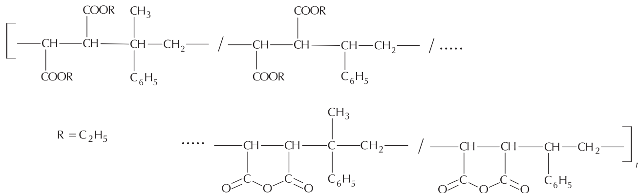
poli[(dietil-fumarat;maleinanhidrid)-alt-(izopropilbenzen;stiren)]
