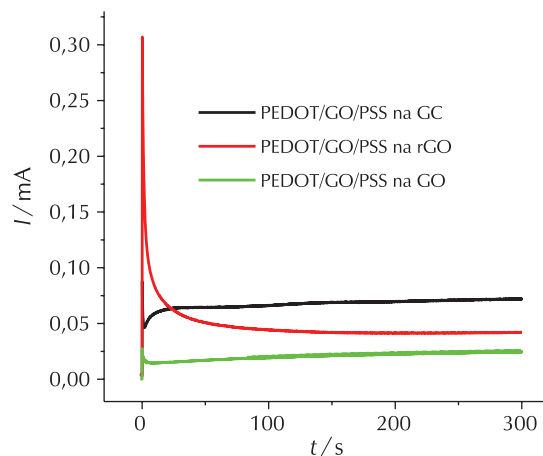
Slika 12 – Kronoamperometrijski odzivi zabilježeni tijekom sinteze PEDOT/GO/PSS slojeva na različitim podlogama pri potencijalu od 1,00 V
